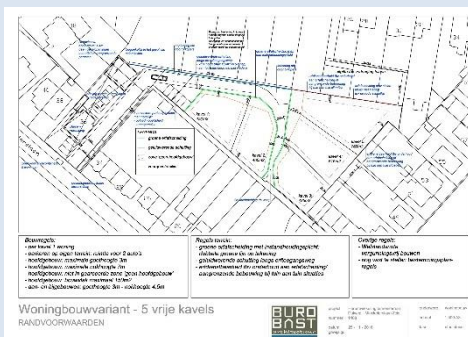
Uitwerking kavelvariant
